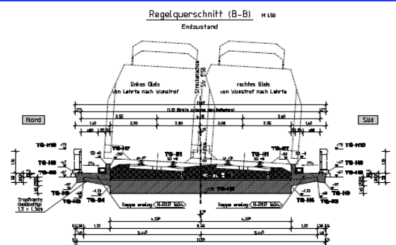
Regelquerschnitt
