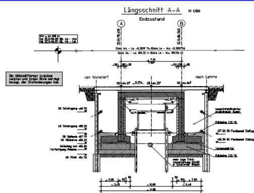
Längsschnitt
