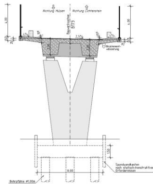
Ansicht Pfeiler (Vorzugsvariante)
