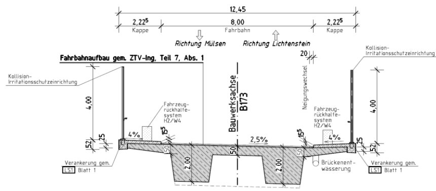
Regelquerschnitt (Vorzugsvariante)
