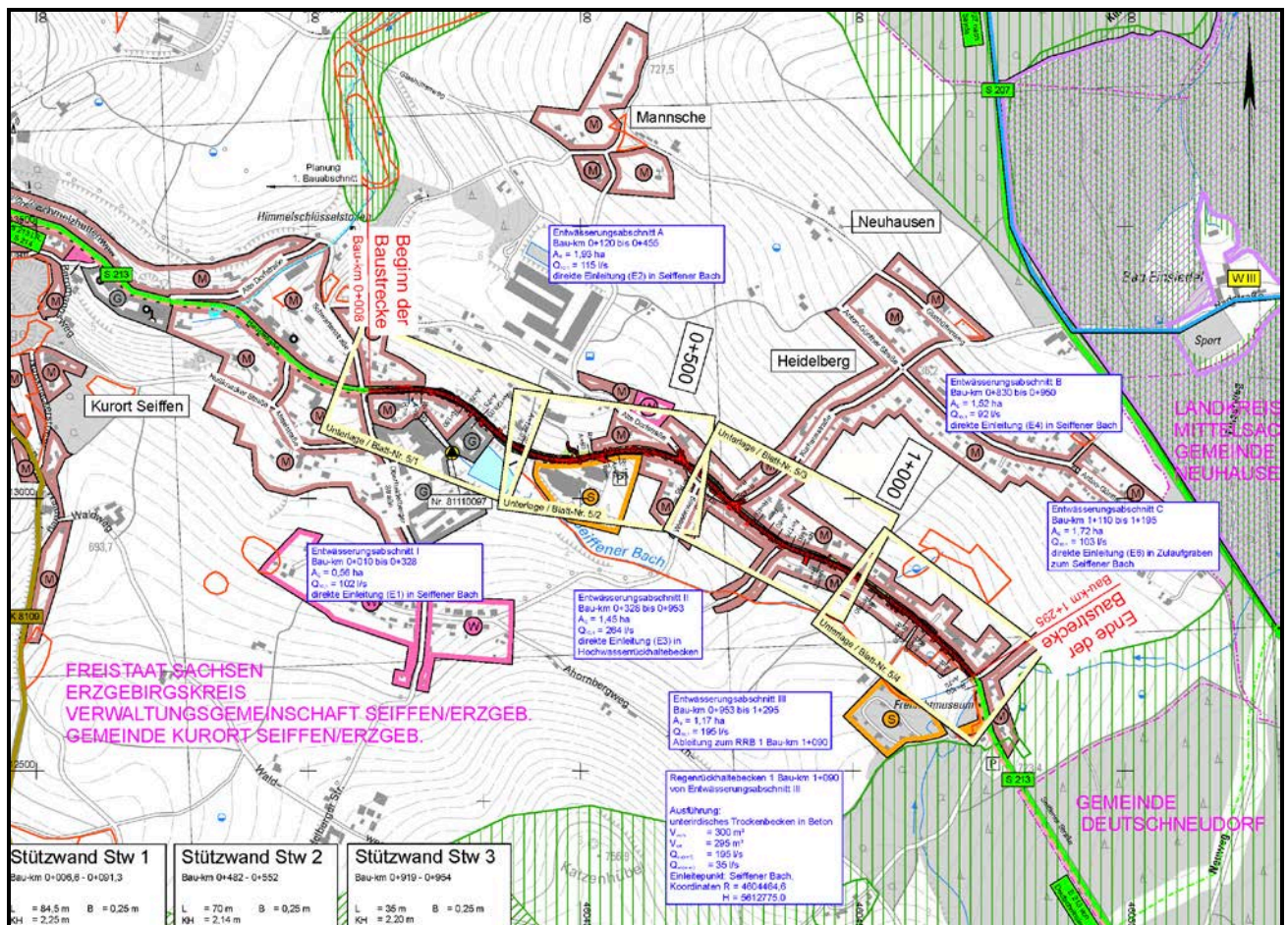
Übersichtsplan
