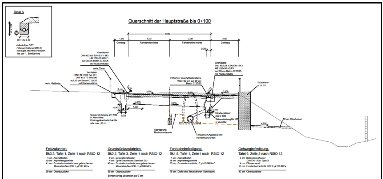
Regelquerschnitt mit Stützwand
