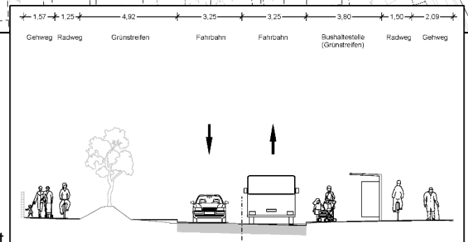
Regelquerschnitt
